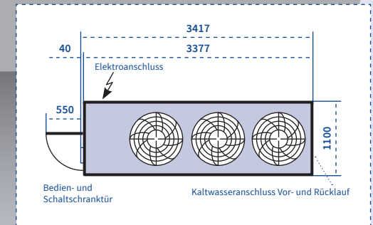
Betriebs- und Serviceabstand umlaufend 1,00 m.
